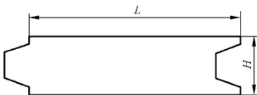
图 3 TG 型产品（榫槽）
